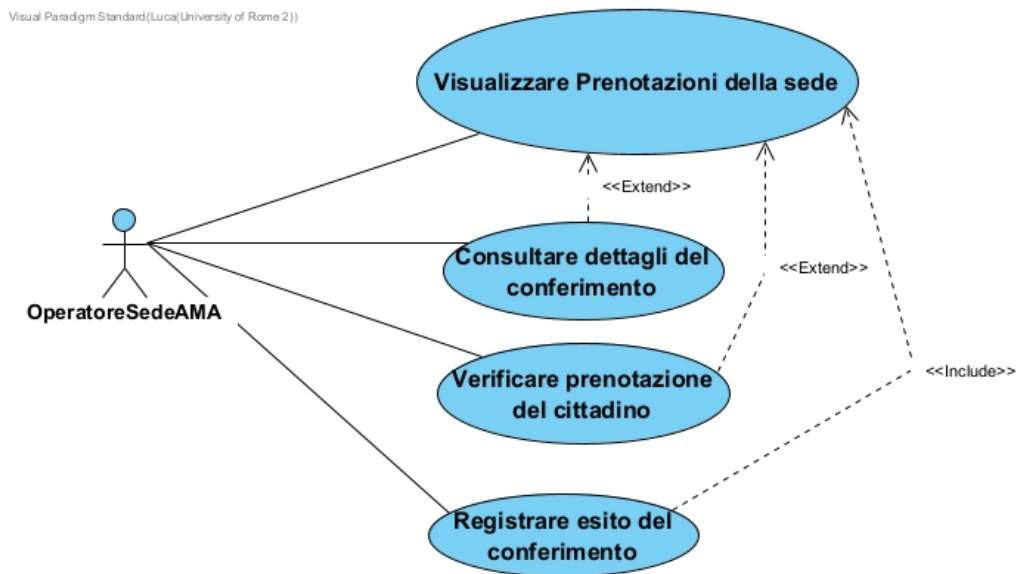
Figura 4: Use Case Diagram — Operatore di sede AMA
