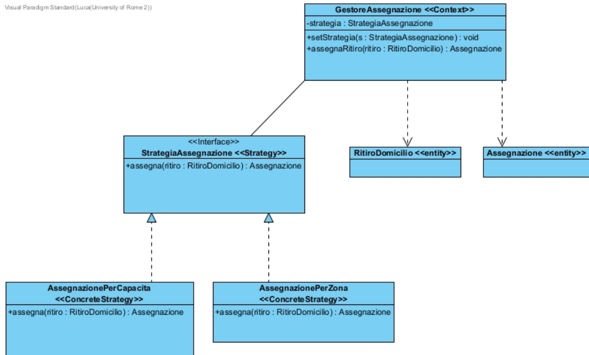
Figura 51: Struttura UML del Design Pattern Strategy applicato a MyAma
